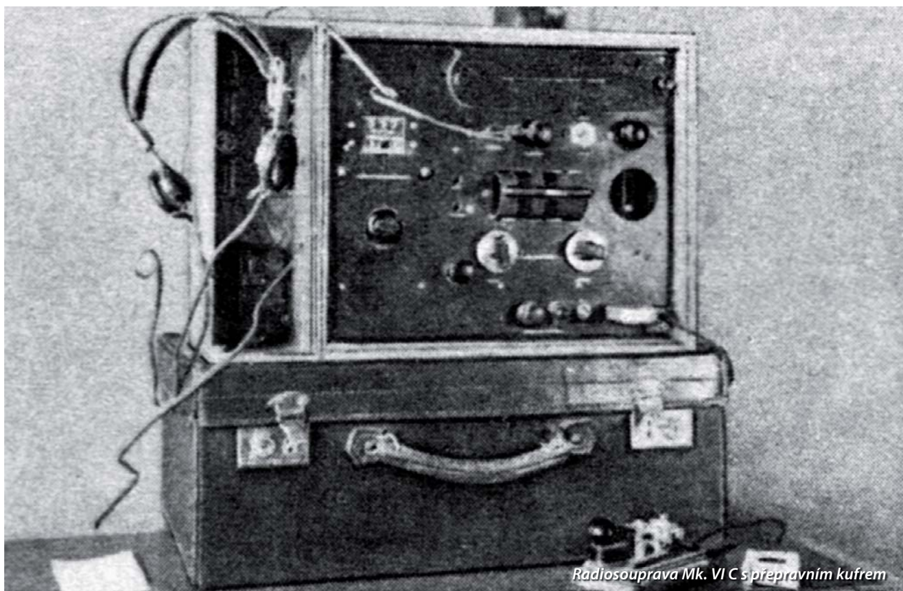
Přijímač Hallicrafters SX24 Sky rider Defiant
